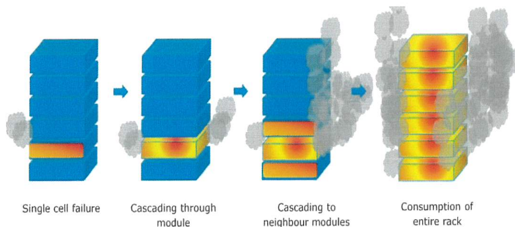
Figura 4 Assenza barriere termiche: Cascading Thermal Runaway
