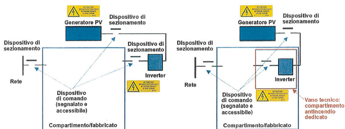
Figura 12 – Esempi di sezionamento di emergenza
